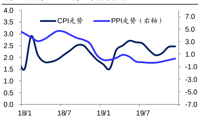
图11 CPI 同比、PPI 同比与预测 (%)
